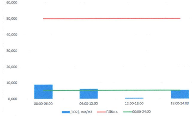
SO₂, мкг/м³
