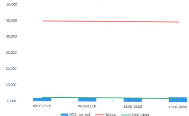
SO₂, мкг/м³
