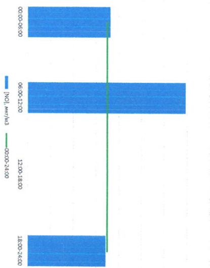
NO, мкг/м³
