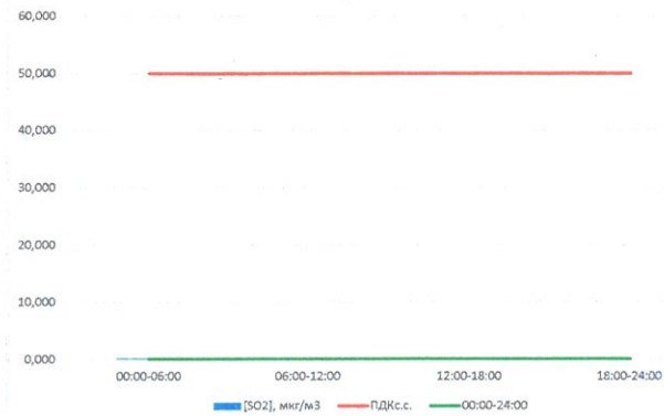
SO 2 , мкг/м³
