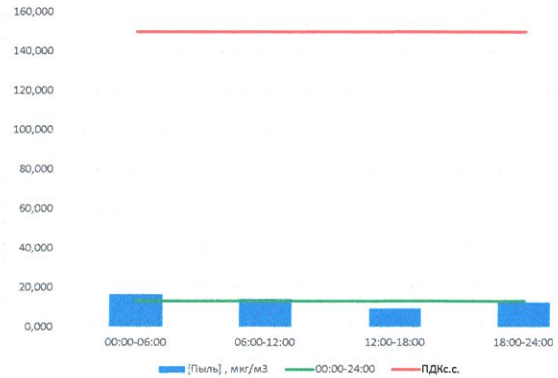
Пыль, мкг/м³
