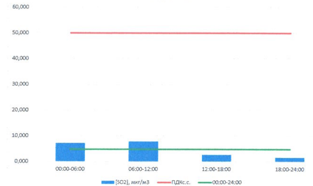
SO2, мкг/м³
