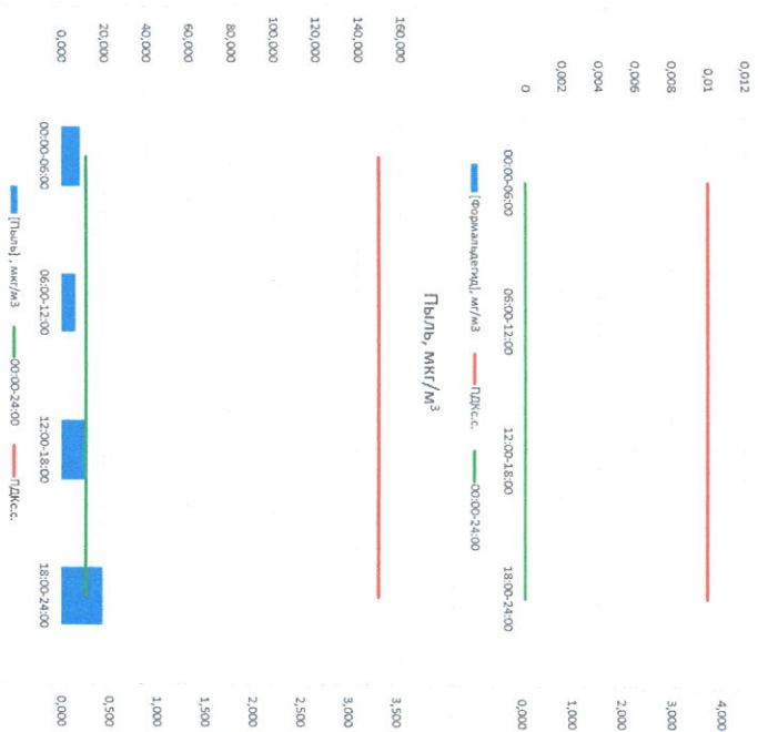
Формальдегид, мкг/м³
