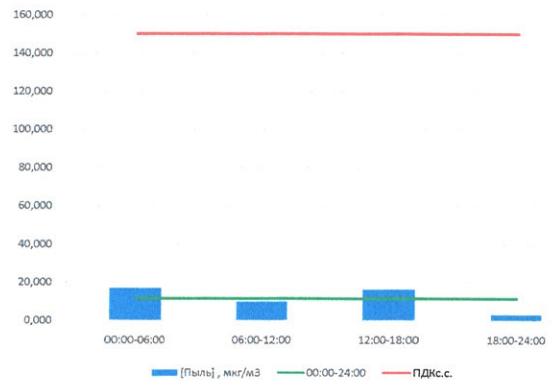
Пыль, мкг/м³
