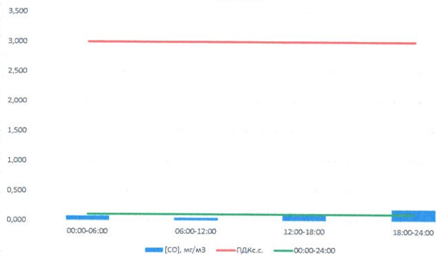
CO, мг/м³
