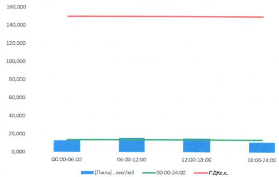
Пыль, мкг/м³
