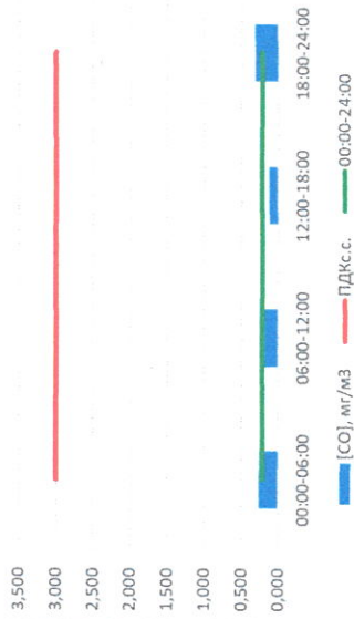
CO, мг/м³
