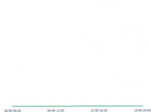
NO, мкг/м³
