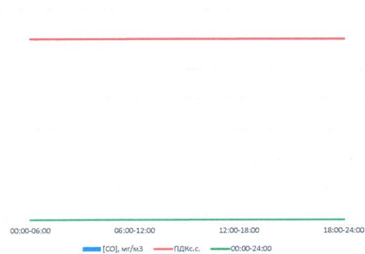
CO, мкг/м³
