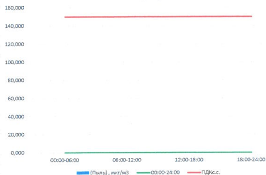
Пыль, мкг/м³
