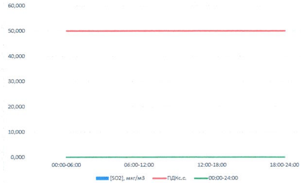
SO 2 , мкг/м³
