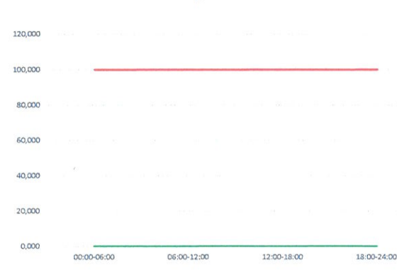
NO 2 , мкг/м³
