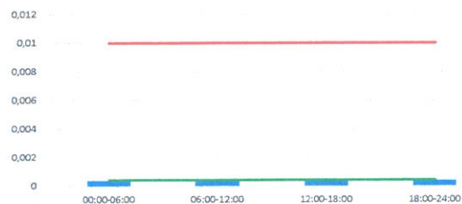
Формальдегид, мг/м³
