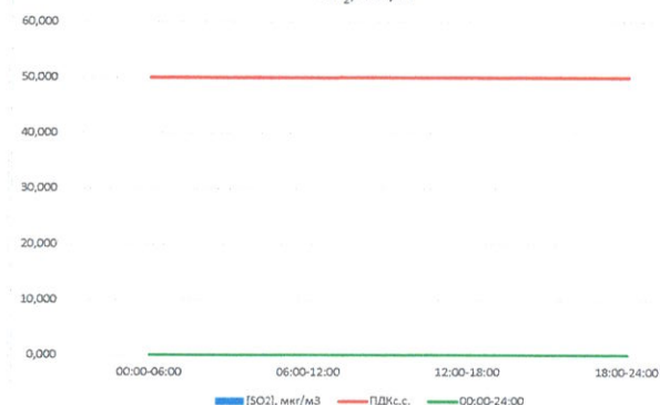
SO 2 , мкг/м³
