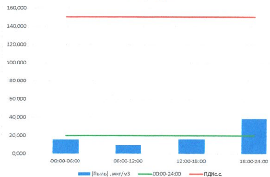
Пыль, мкг/м³
