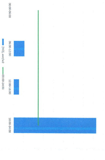
NO, мкг/м³
