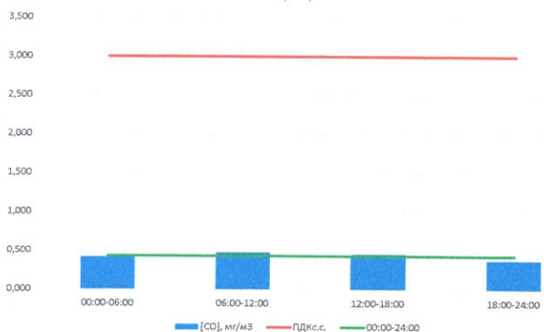
CO, мг/м³
