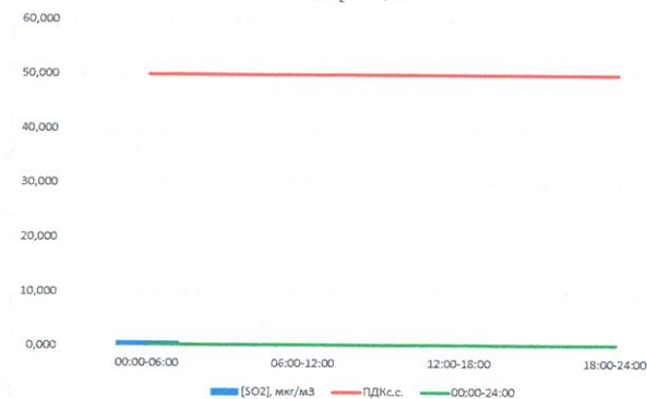
SO 2 , мкг/м³
