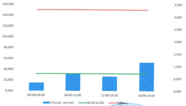
Пыль, мкг/м³
