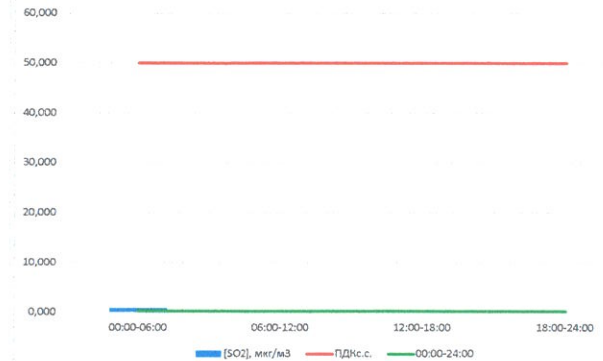
SO 2 , мкг/м³
