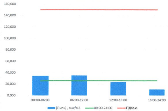
Пыль, мкг/м³
