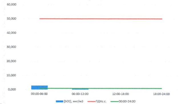
SO 2 , мкг/м³
