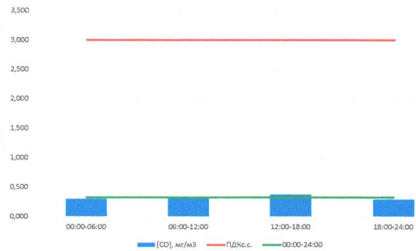
CO, мг/м³
