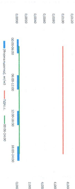
Формальдегид, мкг/м 3
