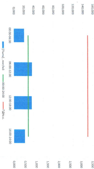
Пыль, мкг/м 3
