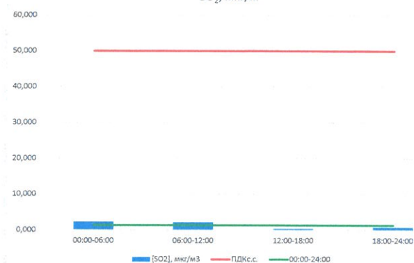
SO 2 , мкг/м³
