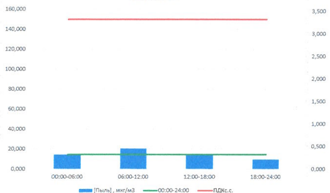
Пыль, мкг/м³
