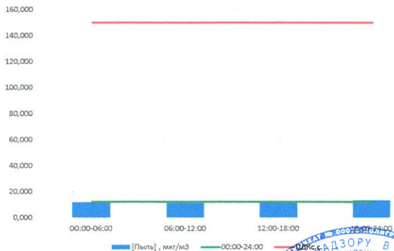
Пыль, мкг/м³
