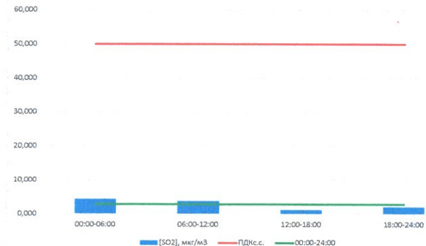
SO2, мкг/м³
