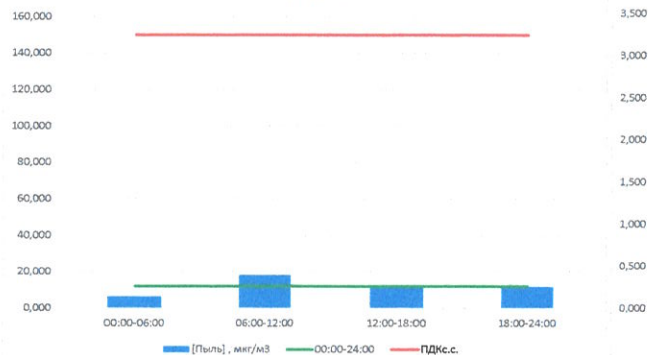
Пыль, мкг/м³
