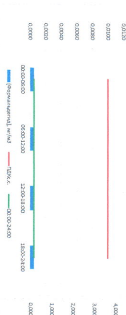
Формальдегид, мкг/м³
