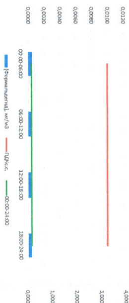
Формальдегид, мкг/м 3
