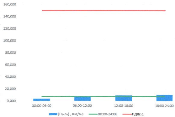
Пыль, мкг/м³
