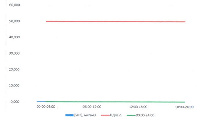
SO 2 , мкг/м³
