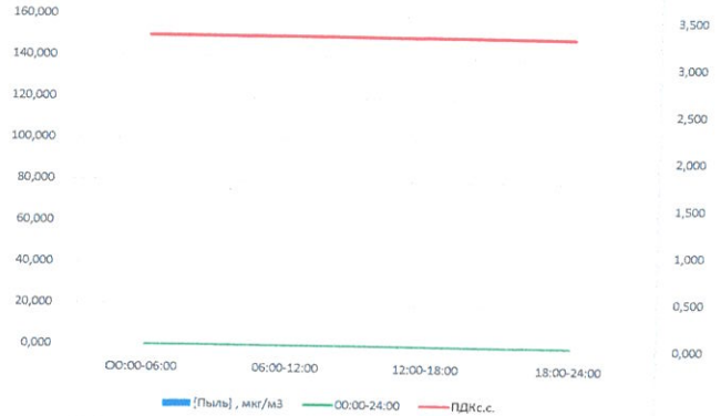
Пыль, мкг/м³
