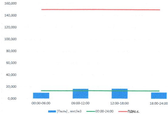
Пыль, мкг/м³
