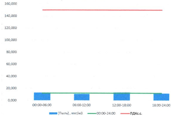
Пыль, мкг/м³
