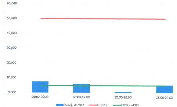
SO 2 , мкг/м³
