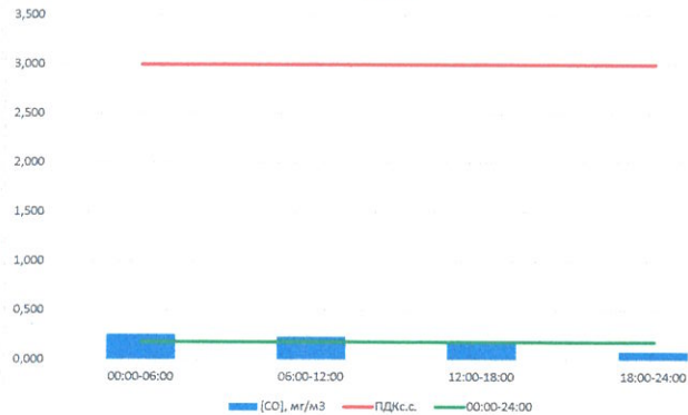
CO, мг/м³
