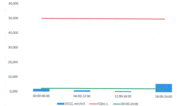
SO2, мкг/м³
